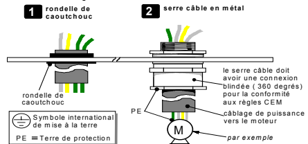
Figure 3-4 Passages et fixation des câbles et écrans
