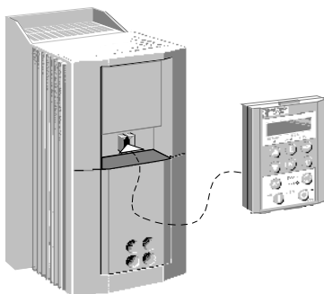
Figure 3-7 Principe de raccordement de la console opérateur 6901
