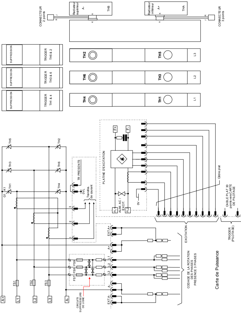
Figure 13-13 Circuit de puissance 4 quadrants – Taille H utilisant AH46001U001
