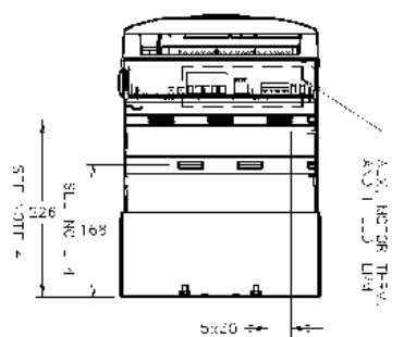
Figure 3-13 Taille 4 Ensemble de puissance 380 - 830A (ref. HG466700U001)
