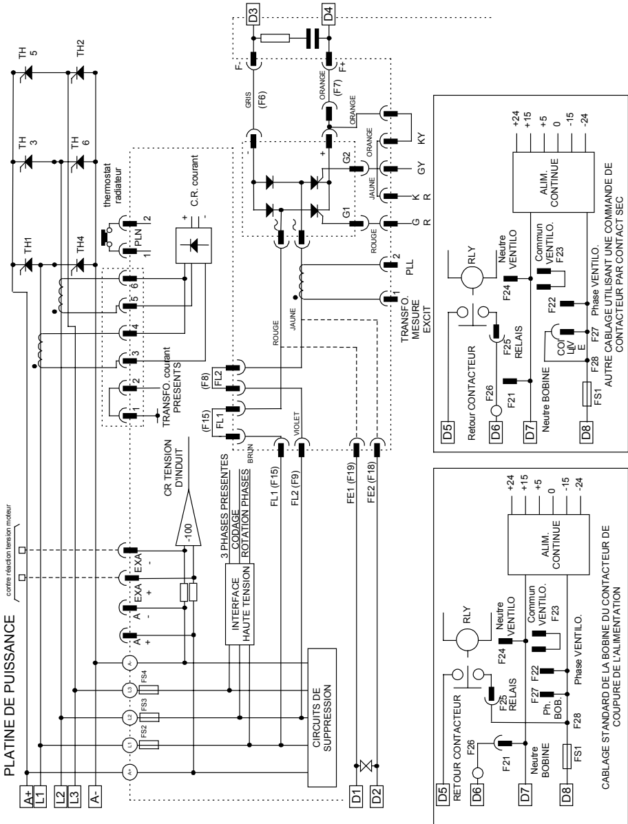
Figure 13-7 Circuit de puissance 2 quadrants - Taille 3 utilisant AH385851U003, U004
